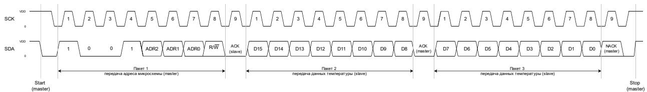
Рисунок 8. Чтение данных температурного кода
