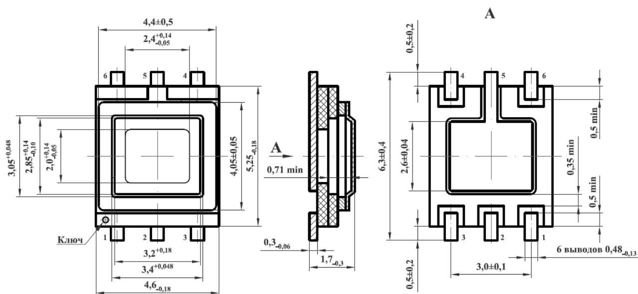
Рисунок 9. Габаритный чертеж корпуса 5221.6-1 (размеры в мм)
