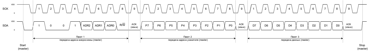
Рисунок 7. Временная диаграмма записи данных
