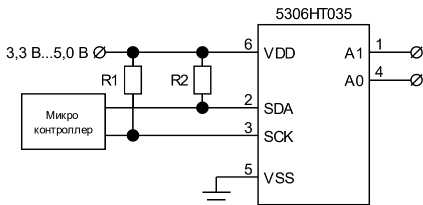
Рисунок 3. Рекомендуемая схема применения
