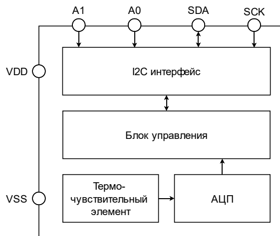
Рисунок 1. Структурная схема
