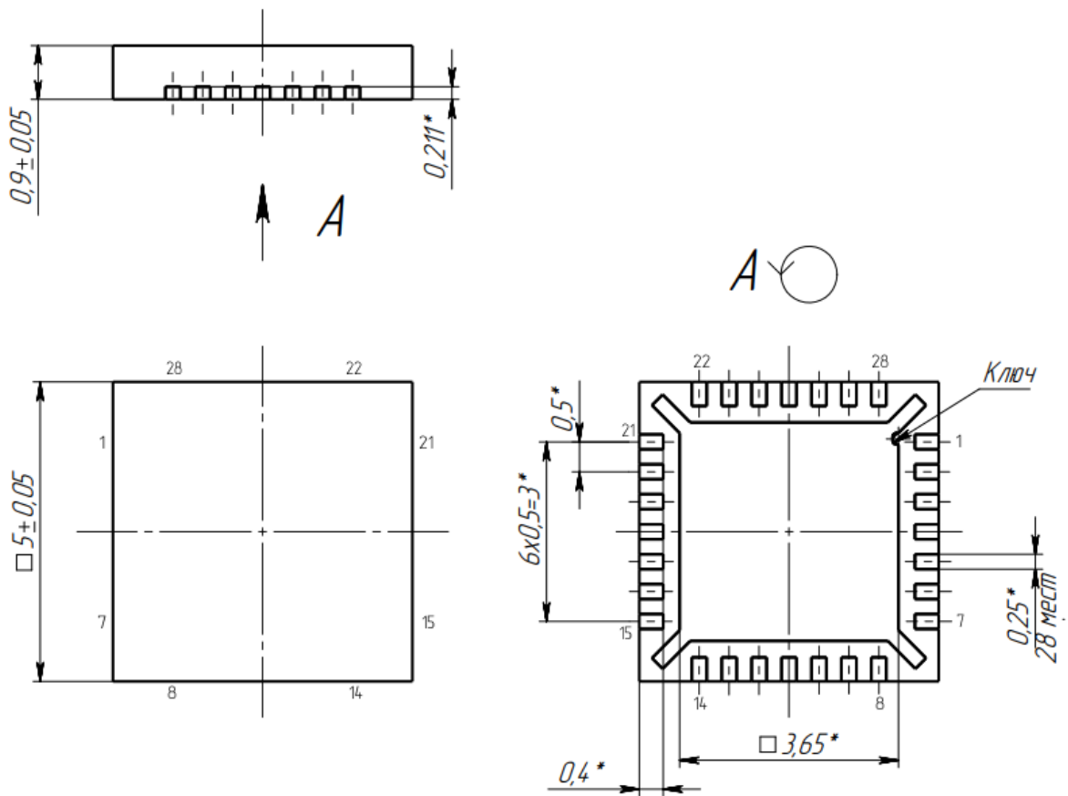
Рисунок 33. Габаритный чертеж корпуса 5102.28-1 К (размеры в мм)
