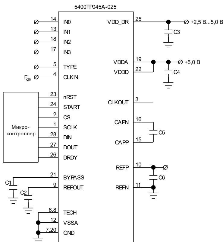
Рисунок 21. Рекомендуемая схема применения при использовании абсолютных измерений (схема с внешним опорным уровнем)
