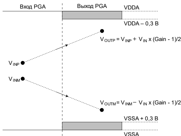
Рисунок 24. Диапазон входа/выхода усилительного каскада
