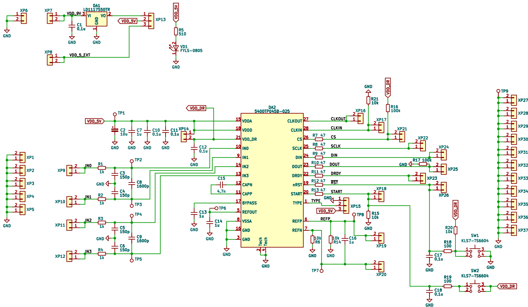
Рисунок 31. Электрическая схема демонстрационной платы КФЦС.441461.230 для микросхемы 5400TP045B-025
