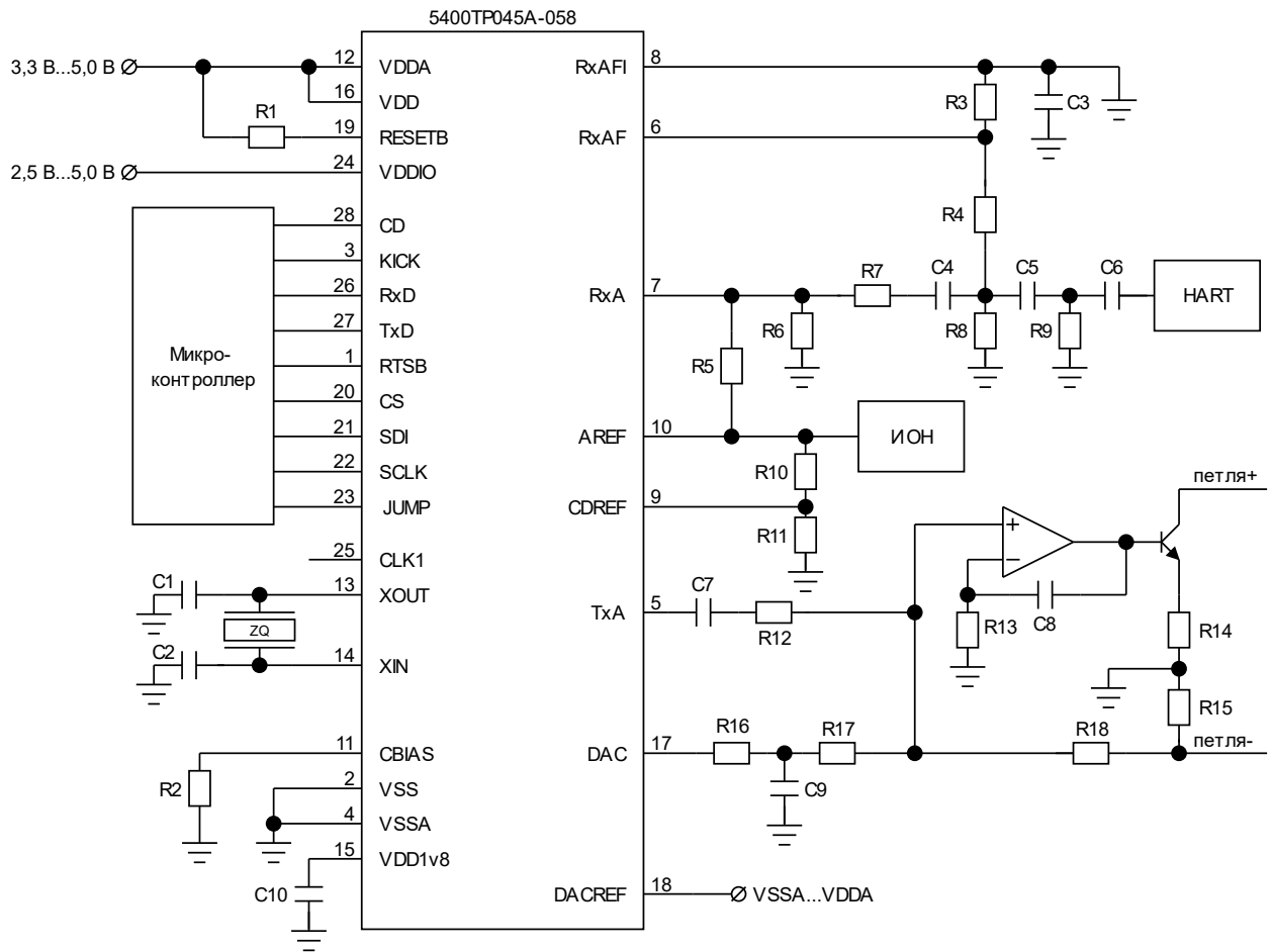
Рисунок 4. Рекомендуемая схема применения
