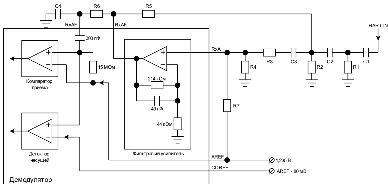
Рисунок 10. Внешние пассивные элементы для входного фильтра
