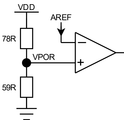
Рисунок 14. Структурная схема блока сброса
