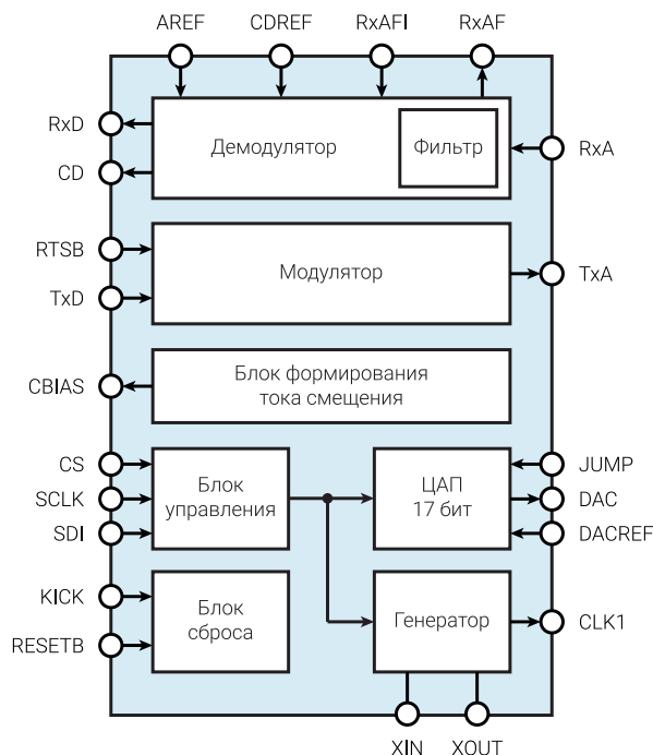
Рисунок 1. Структурная схема
