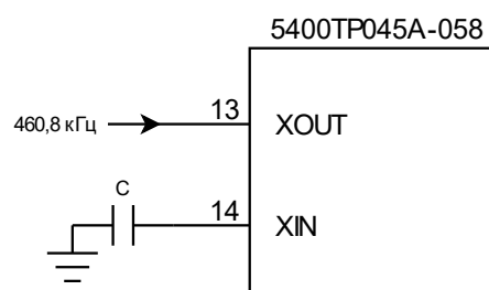
Рисунок 13. Генератор с внешним тактовым сигналом
