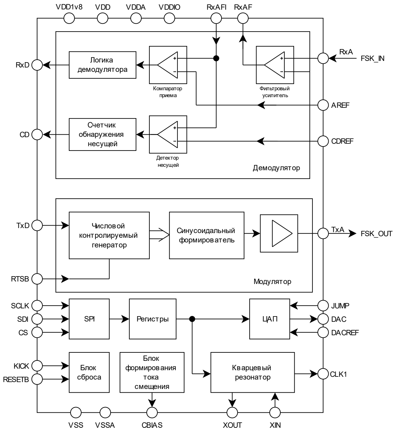
Рисунок 6. Блок схема 5400TP045A-058
