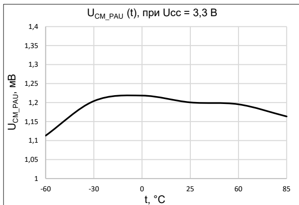
Рисунок 3. Зависимость напряжения смещения блока PAU от температуры (при U сс = 3,3 В)
