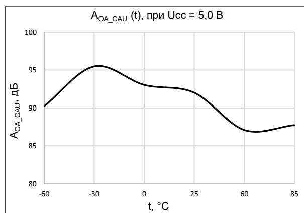
Рисунок 12. Зависимость коэффициента усиления блока CAU от температуры (при U_{CC} = 5,0 В)
