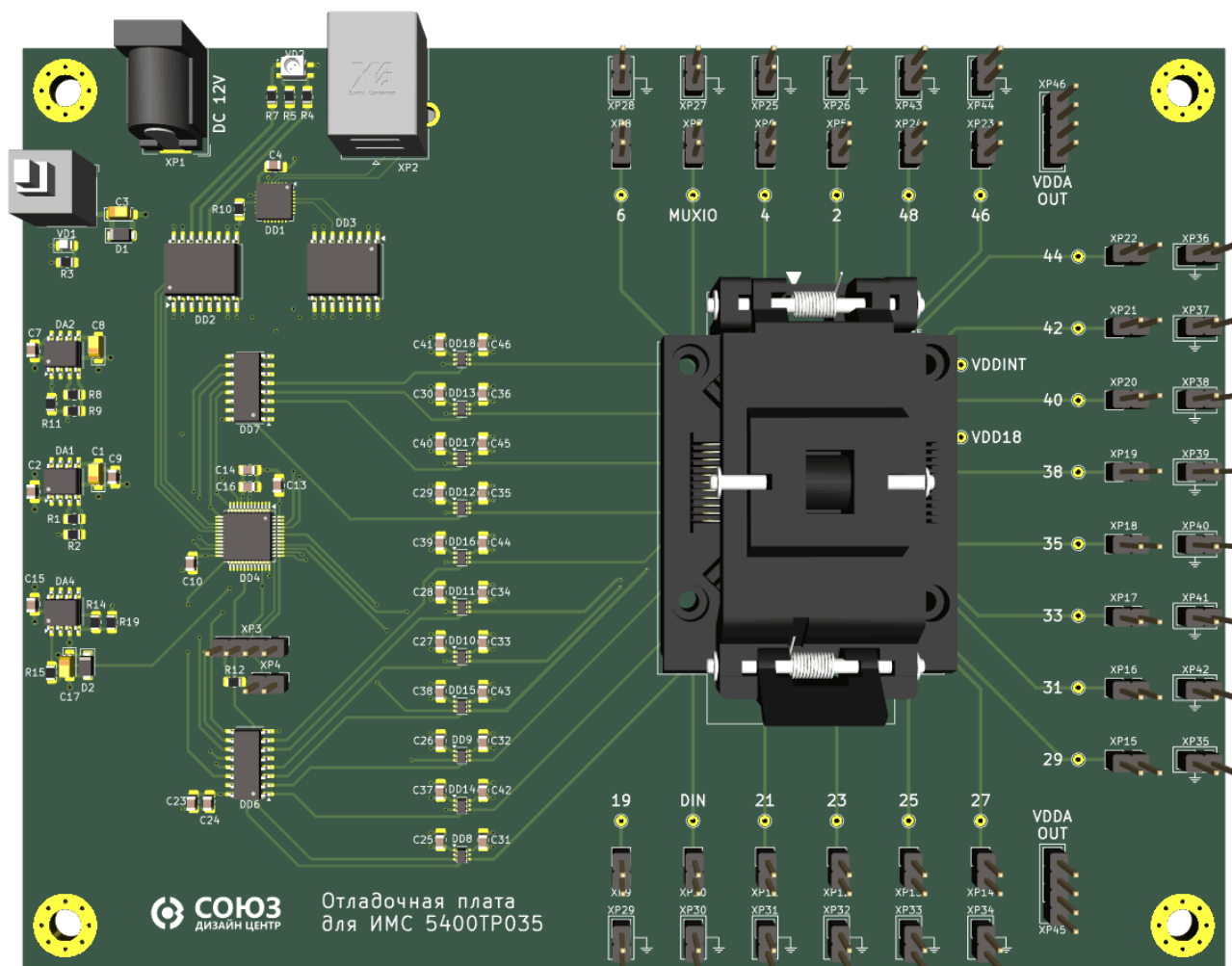
Рисунок 32. Отладочная плата КФЦС.441461.279
