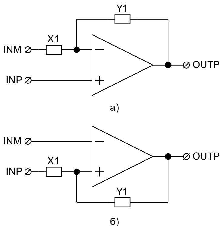
Рисунок 29. Эквивалентная схема потенциометров в блоке CAU: а) отрицательная обратная связь; б) положительная обратная связь
