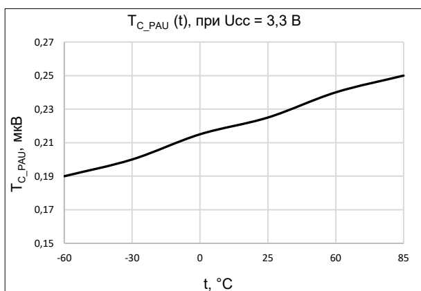
Рисунок 7. Зависимость задержки переключения компаратора блока PAU от температуры (при U сс = 3,3 В)
