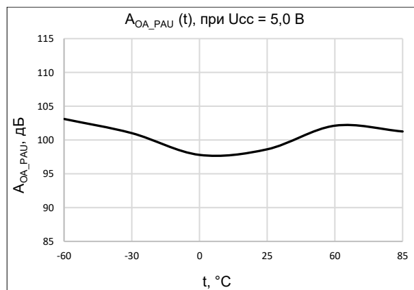
Рисунок 6. Зависимость коэффициента усиления блока PAU от температуры (при U сс = 5,0 В)
