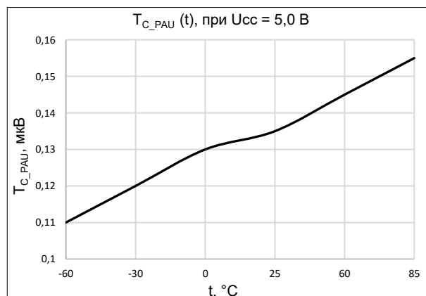
Рисунок 8. Зависимость задержки переключения компаратора блока PAU от температуры (при U сс = 5,0 В)
