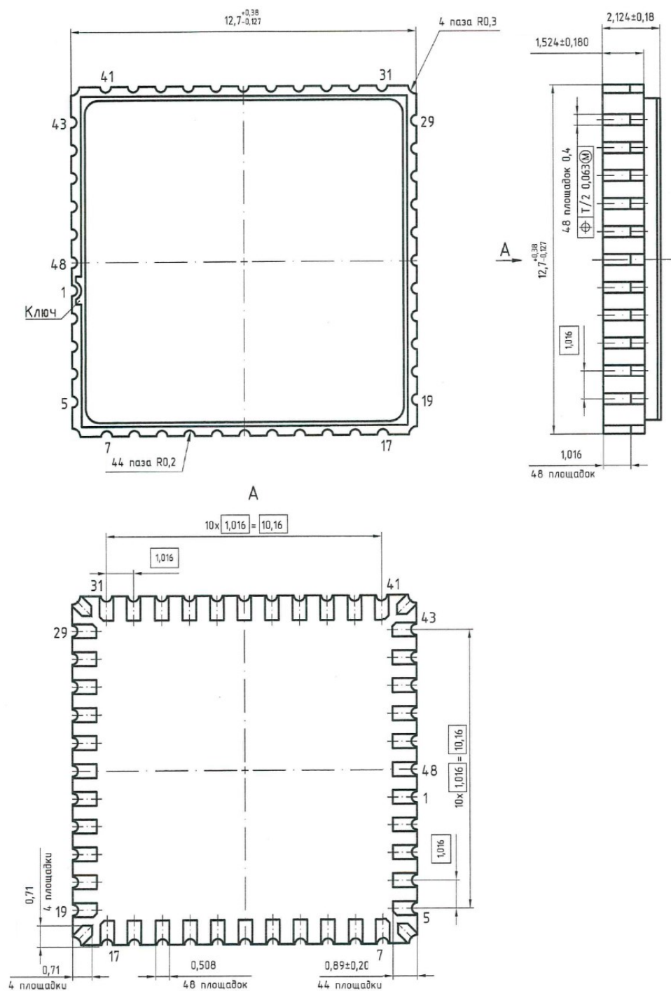
Рисунок 33. Габаритный чертеж корпуса 5142.48-А (размеры в мм)
