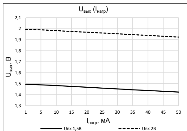
Рисунок 22. Зависимость выходного напряжения аналогового буфера от тока нагрузки (при входном напряжении 1,5 В и 2,0 В)
