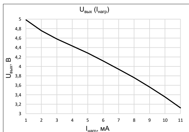
Рисунок 26. Зависимость выходного напряжения цифрового буфера от тока нагрузки
