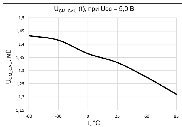
Рисунок 10. Зависимость напряжения смещения блока CAU от температуры (при U_{CC} = 5,0 В)
