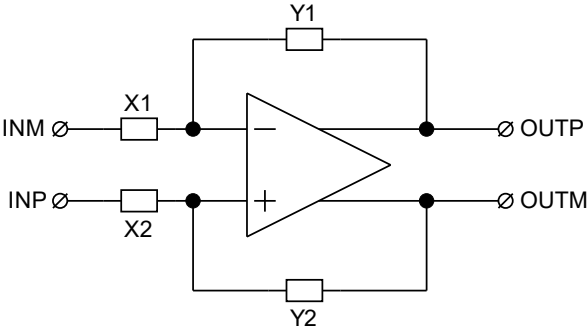
Рисунок 28. Эквивалентная схема потенциометров в блоке PAU
