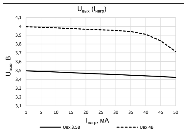
Рисунок 24. Зависимость выходного напряжения аналогового буфера от тока нагрузки (при входном напряжении 3,5 В и 4,0 В)
