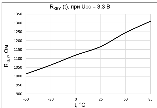
Рисунок 15. Зависимость сопротивления коммутационного ключа от температуры (при U_{СС} = 3,3 В)
