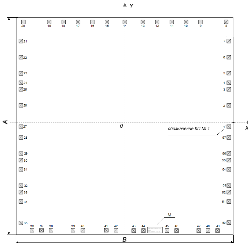
Рисунок 34. Габаритный чертеж кристалла 5400TP03H4
