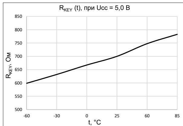
Рисунок 16. Зависимость сопротивления коммутационного ключа от температуры (при U_{СС} = 5,0 В)
