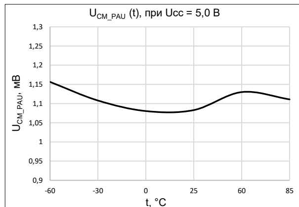
Рисунок 4. Зависимость напряжения смещения блока PAU от температуры (при U сс = 5,0 В)
