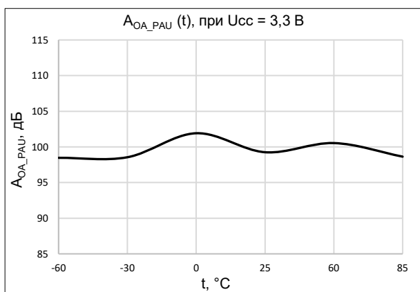
Рисунок 5. Зависимость коэффициента усиления блока PAU от температуры (при U сс = 3,3 В)
