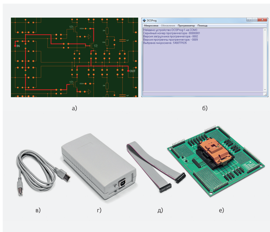
Рис.2. Отладочный комплект микросхемы 5400TP035: а) интерфейс САПР; б) интерфейс ПО программатора; в-д) элементы программатора; е) макетная плата
