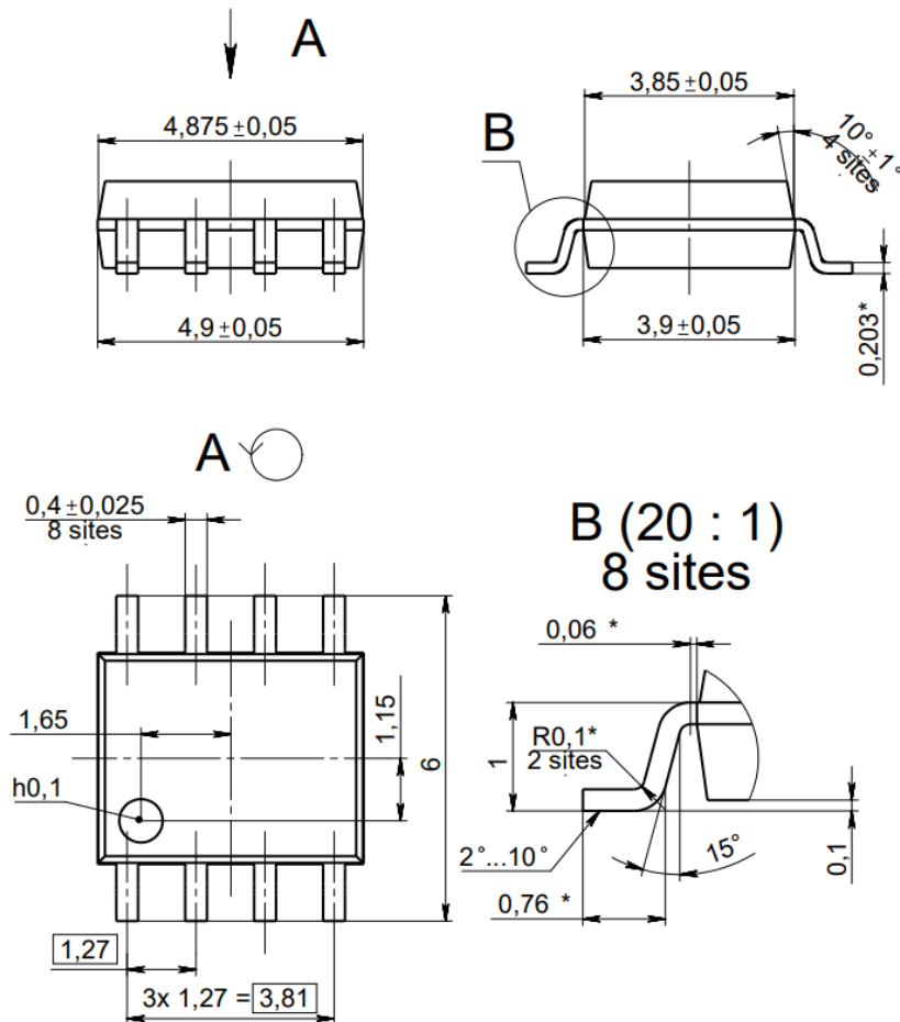
Рисунок 19. Габаритный чертеж корпуса 4341.6-1 К (размеры в мм)
