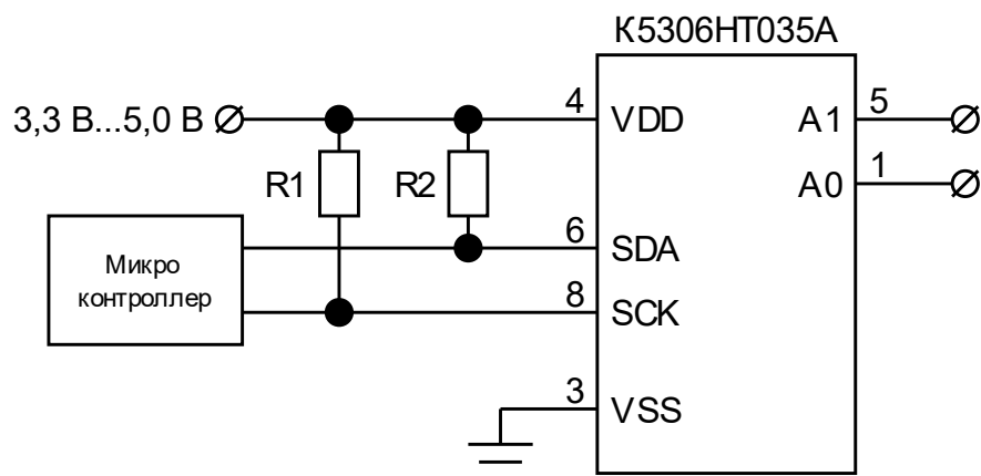
Рисунок 11. Рекомендуемая схема применения для микросхемы K5306HT035A
