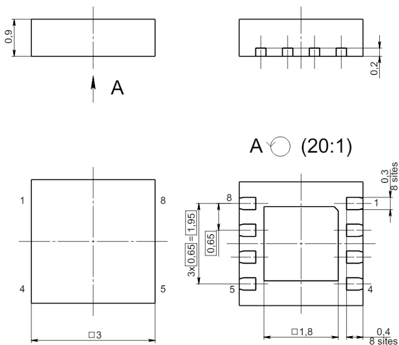
Рисунок 20. Габаритный чертеж корпуса 5241.8-1H3 К (размеры в мм)
