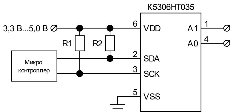
Рисунок 10. Рекомендуемая схема применения для микросхемы K5306HT035
