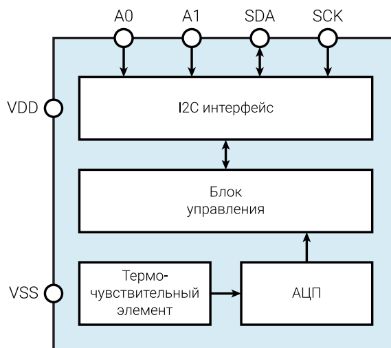
Рисунок 1. Структурная схема
