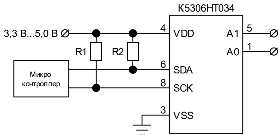
Рисунок 9. Рекомендуемая схема применения для микросхемы K5306HT034
