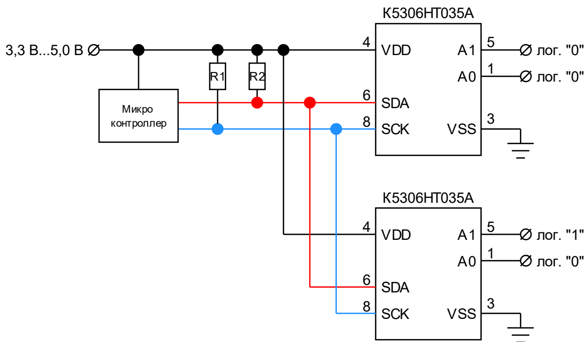
Рисунок 12. Схема применения нескольких микросхем на линии (на примере K5306HT035A)
