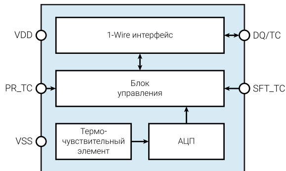
Рисунок 1. Структурная схема
