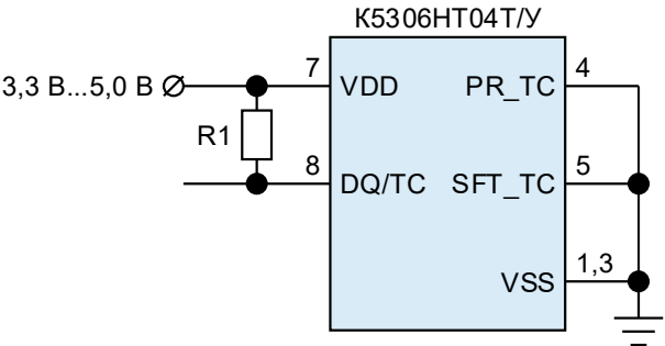
Рисунок 7. Рекомендуемая схема применения для микросхемы K5306HT04T/Y
