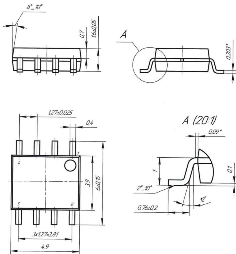
Рисунок 18. Габаритный чертеж корпуса 4303.8-DH3 К (размеры в мм)
